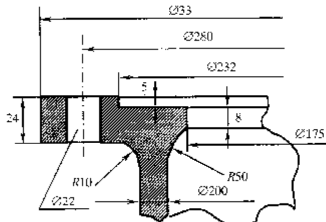
Рисунок Б.24 — Пожарная подставка раструбная
