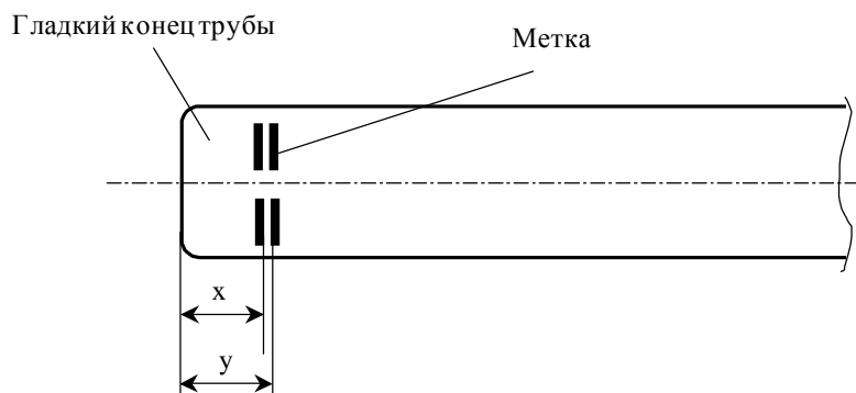
Рисунок 5.8 — Нанесение меток. Метка y равна глубине раструба, а x = y - 10 мм, для всех диаметров труб
