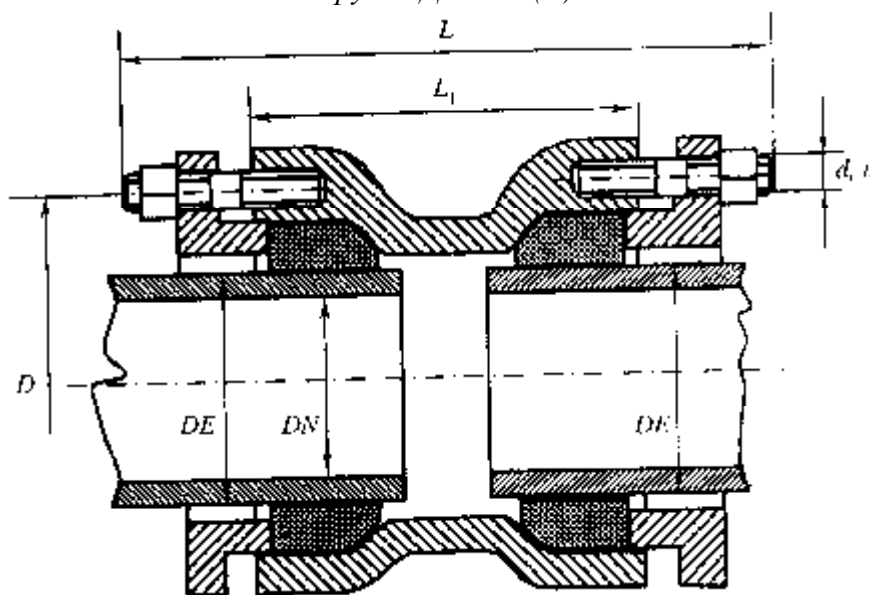
Рисунок Б.21 — Двойной раструб компенсационный
