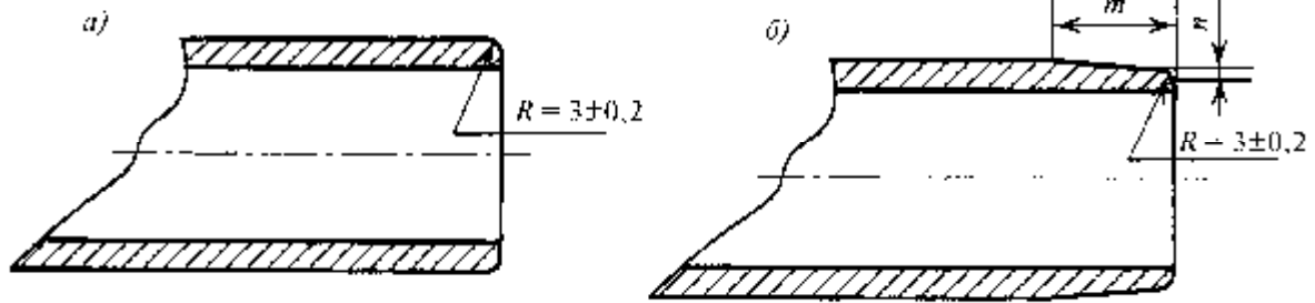
Рисунок А.5 — Торцы гладкого конца трубы
