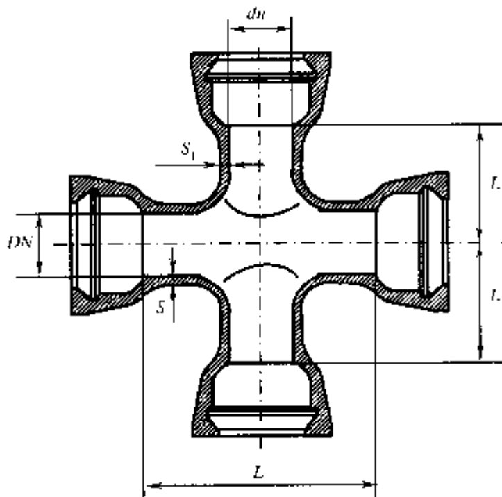
Рисунок Б.28 — Крест раструбный
