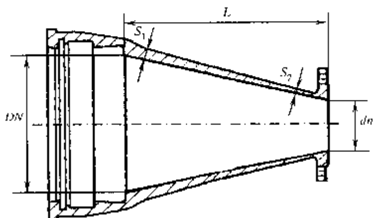
Рисунок Б.14 — Переходраструб — фланец
