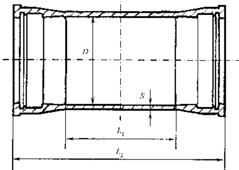
Рисунок Б.33 — Муфта надвижная
