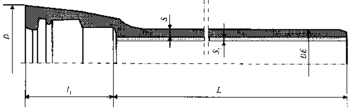
Рисунок А.1 — Труба раструбная под соединение «TYTON»
