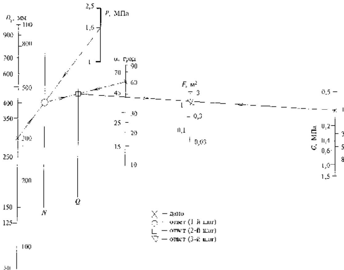
Рисунок 5.10 — Номограмма для выбора опорной площади упоров F на напорном трубопроводе условным диаметром D_n из труб из высокопрочного чугуна с шаровидным графитом с раструбными соединениями, находящиеся под внутренним давлением P , при угле поворота трассы \alpha с опорой на грунт прочностью G ( N и Q — промежуточные шкалы)
