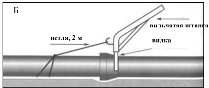
б) при помощи петли и вилчатой штанги
