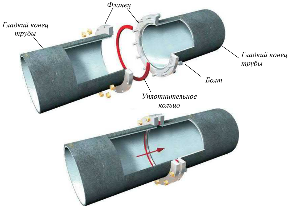
Рисунок 2.12 Фланцевое соединение.
