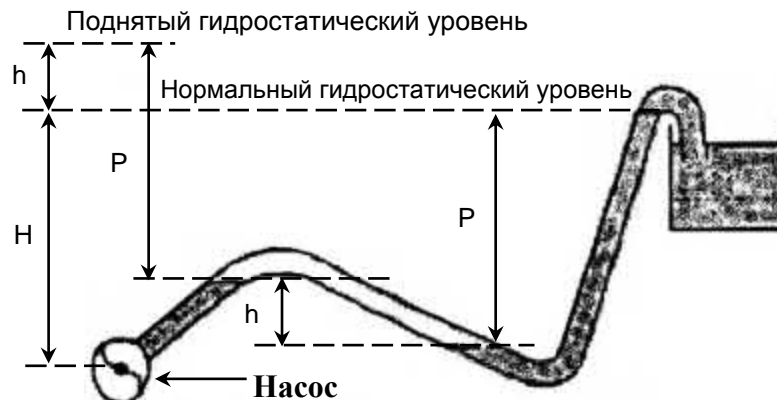
Рисунок 5.4 Условия в напорном трубопроводе.
