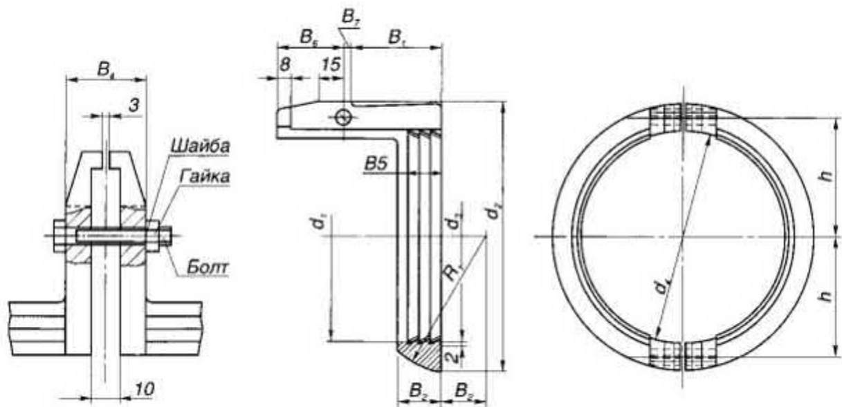
Рисунок 6.11 Стяжное кольцо.
