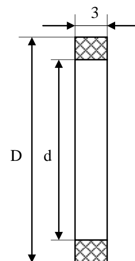
Рисунок 2.15 Уплотнительное кольцо для фланцевого соединения.
