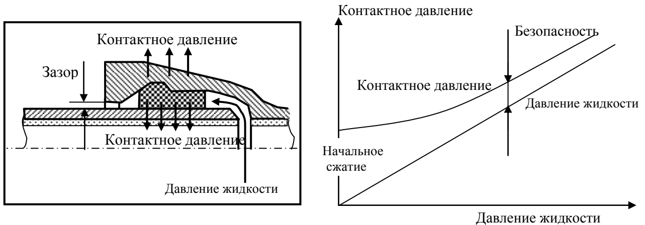
Рисунок 2.16 Контактное давление.
