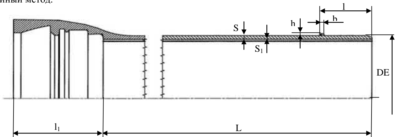
Рисунок 2.10 Труба раструбная с соединением «RJS».
